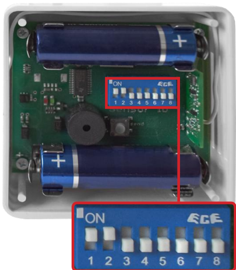
Abb. 3.5.2: Luftbefeuchter codieren
